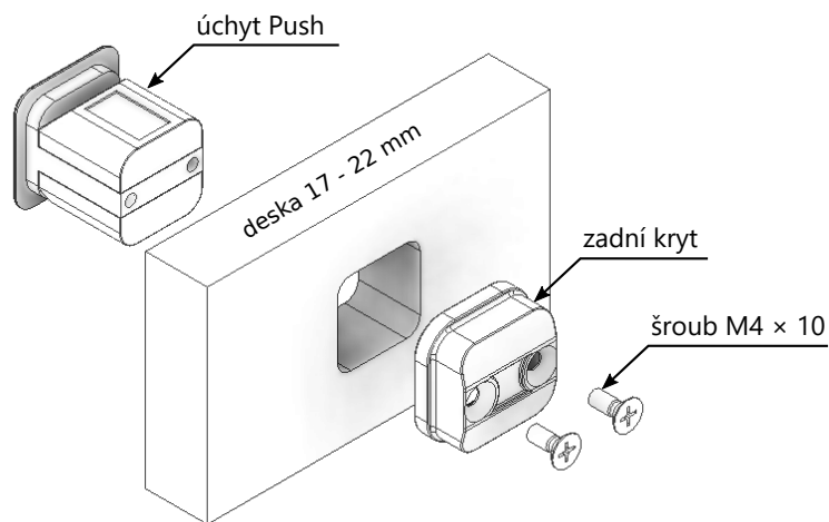
montáž A
