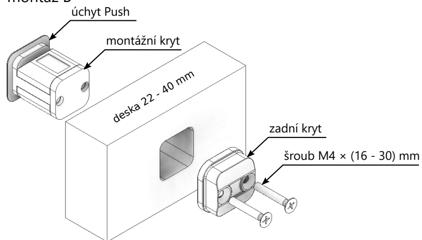
montáž B
