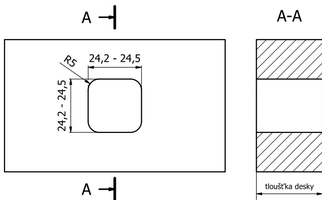
frézování desky
